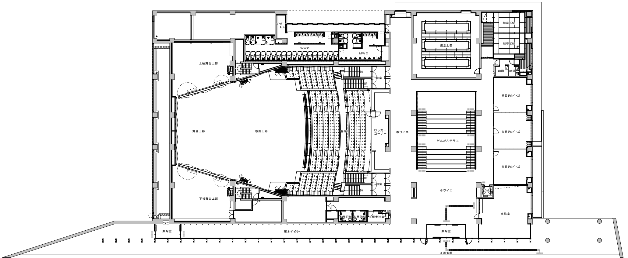
2階平面図
